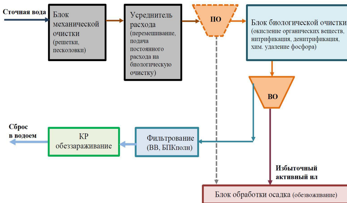
Рис. 4 Блок-схема построения очистных сооружений хозяйственно-бытовых сточных вод муниципального округа Сокольский ВО – вторичный отстойник, ПО – первичный отстойник, КР – УФ обеззараживание
